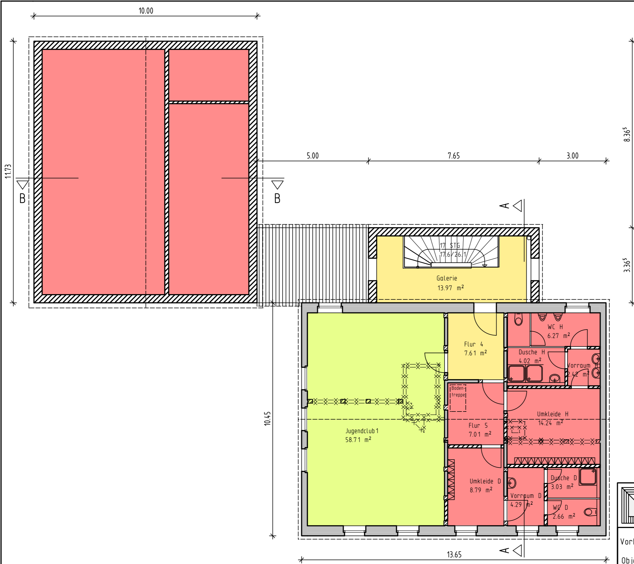
Grundriss Obergeschoss
